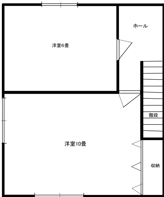
リバーサイドⅢ-E号室 2階改修後間取図
